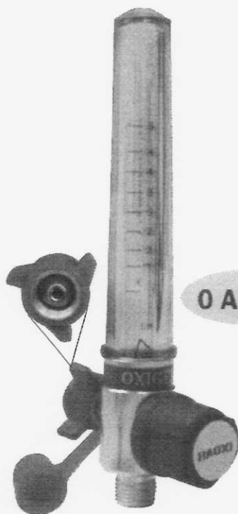
FL 2403 0 A 3 L/MIN P/ AR COMPRIMIDO FL 2407 0 A 3 L/MIN P/ OXIGÊNIO
