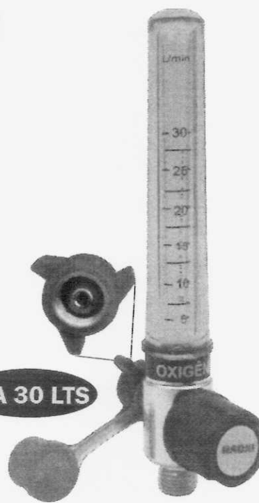
FL 2411 0 A 30 L/MIN P/ AR COMPRIMIDO FL 2412 0 A 30 L/MIN P/ OXIGÊNIO
