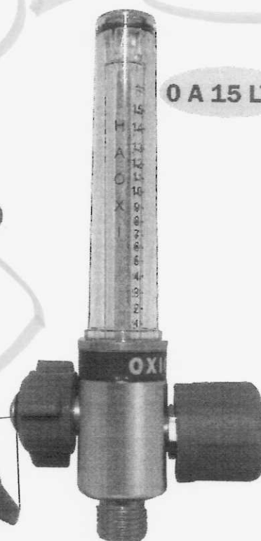
FL 2401 0 A 15 L/MIN P/ OXIGÊNIO
