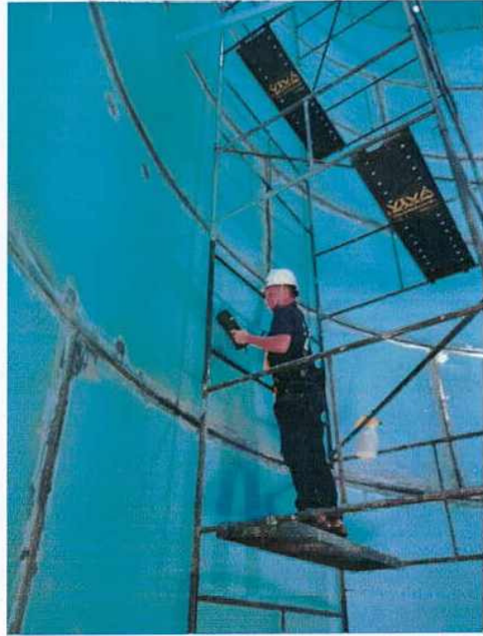
Ultrassom
