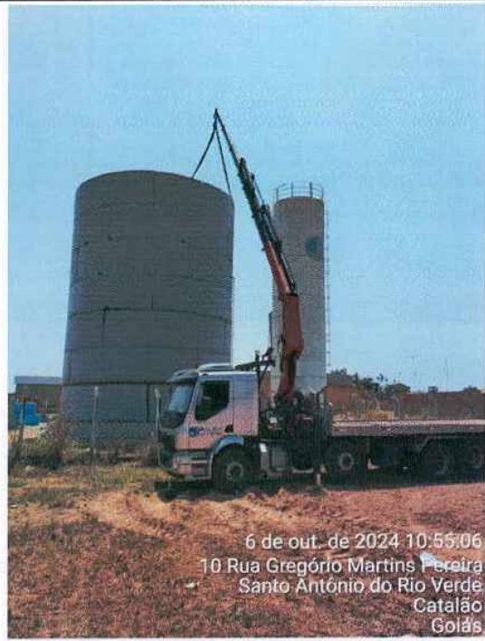
Montagem - Costado
