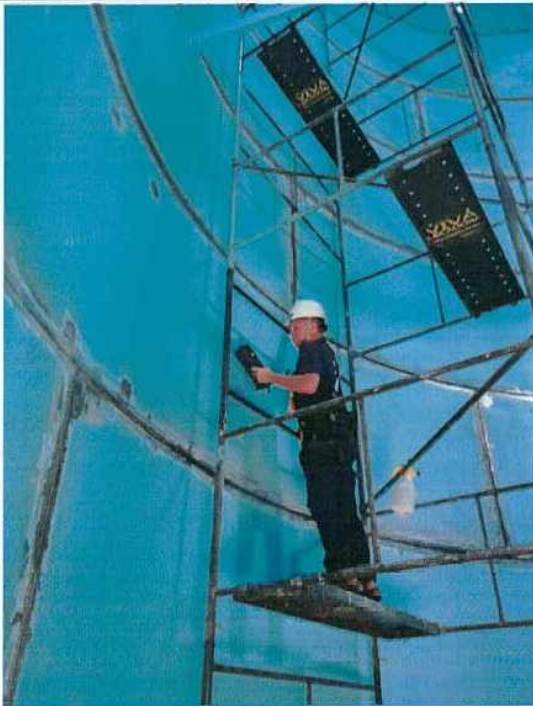
Ultrassom
