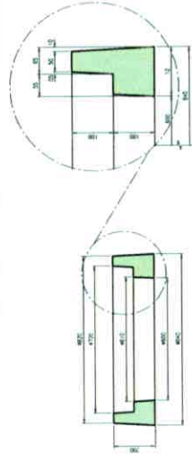
Detalhe do Tampo em Concreto Armado - ESC. 1:10
