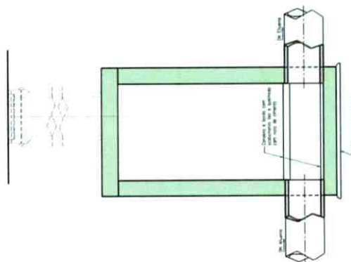
CORTE LONGITUDINAL - ESC. 1:25 (Típico)
