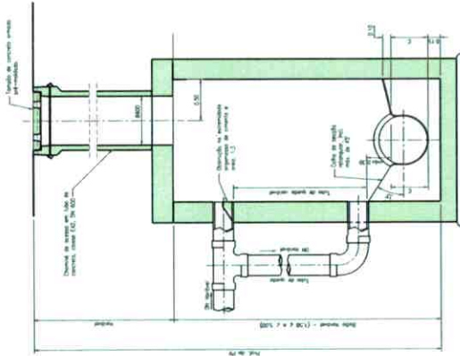
CORTE NO TUBO DE ODEIA - ESC. 1:25 (Típico)
