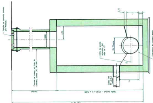
CORTE NA ODEIA LAME - ESC. 1:25 (Típico)
